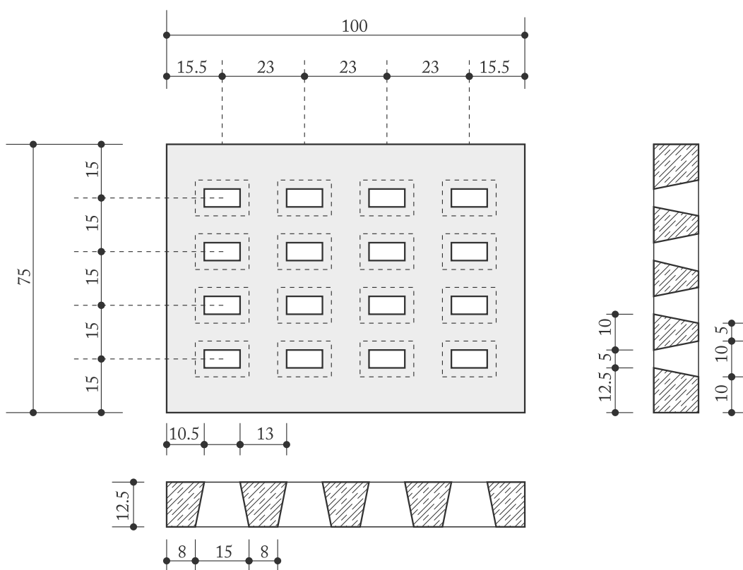
PŁYTA DROGOWA-100x75
