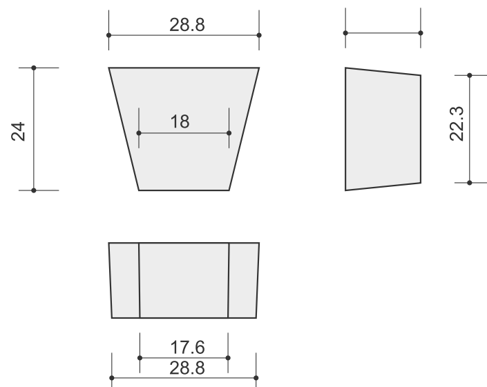
DYBEL POŁÓWKOWY DP-15
