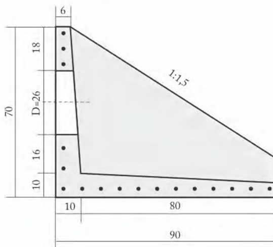
PRZEKRÓJ PODŁUŻNY
